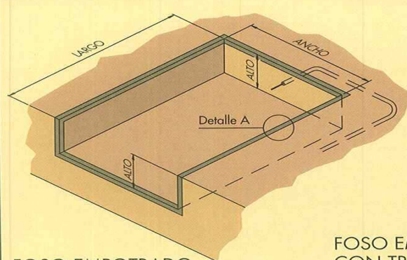
FOSO EMPOTRADO
