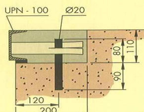
DETALLE B
