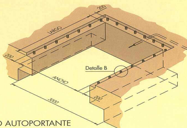
FOSO EMPOTRADO CON TRAMPILLA
