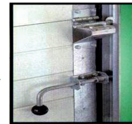
CERROJO Y ESCUADRA Detalle del cerrojo y de las bisagras laterales
